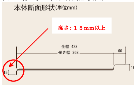
図 2 (参考：本体断面形状図)
